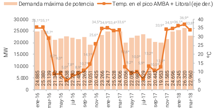
Figura 27. Demanda máxima de potencia y temperatura en el pico 2017-2018, en MW y °C
